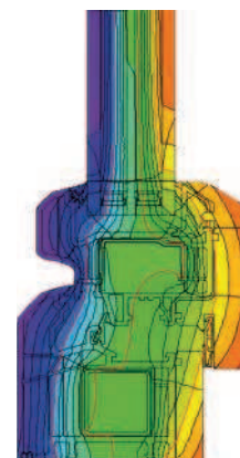
Portoncino CLIMA Wood Sistema a tre guarnizioni PVC-Legno
